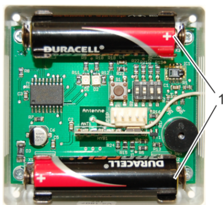
Fig. 12: Insert batteries
