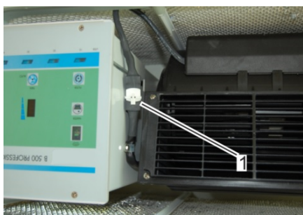
Fig. 56: Connect fan
