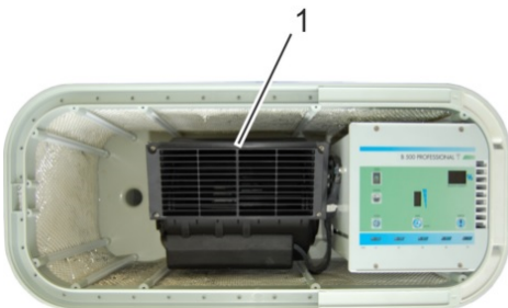
Fig. 42: Vacuum fan
